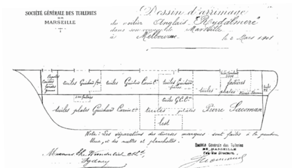
איור 11 - סקיצת חתך ספינה שפירסם קואופרטיב המפעלים במרסיי, ובה מתוארים סוגי סחורה מיצרנים שונים, ביניהם רעפים [Raïter, 1989, עמ' 212]
