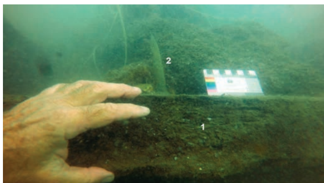
איור 3 - לוח דופן הספינה (עובי: כ-10 ס"מ) [1]; מסמר ברונזה שחיבר את לוח הציפוי לצלעות הספינה [2]
