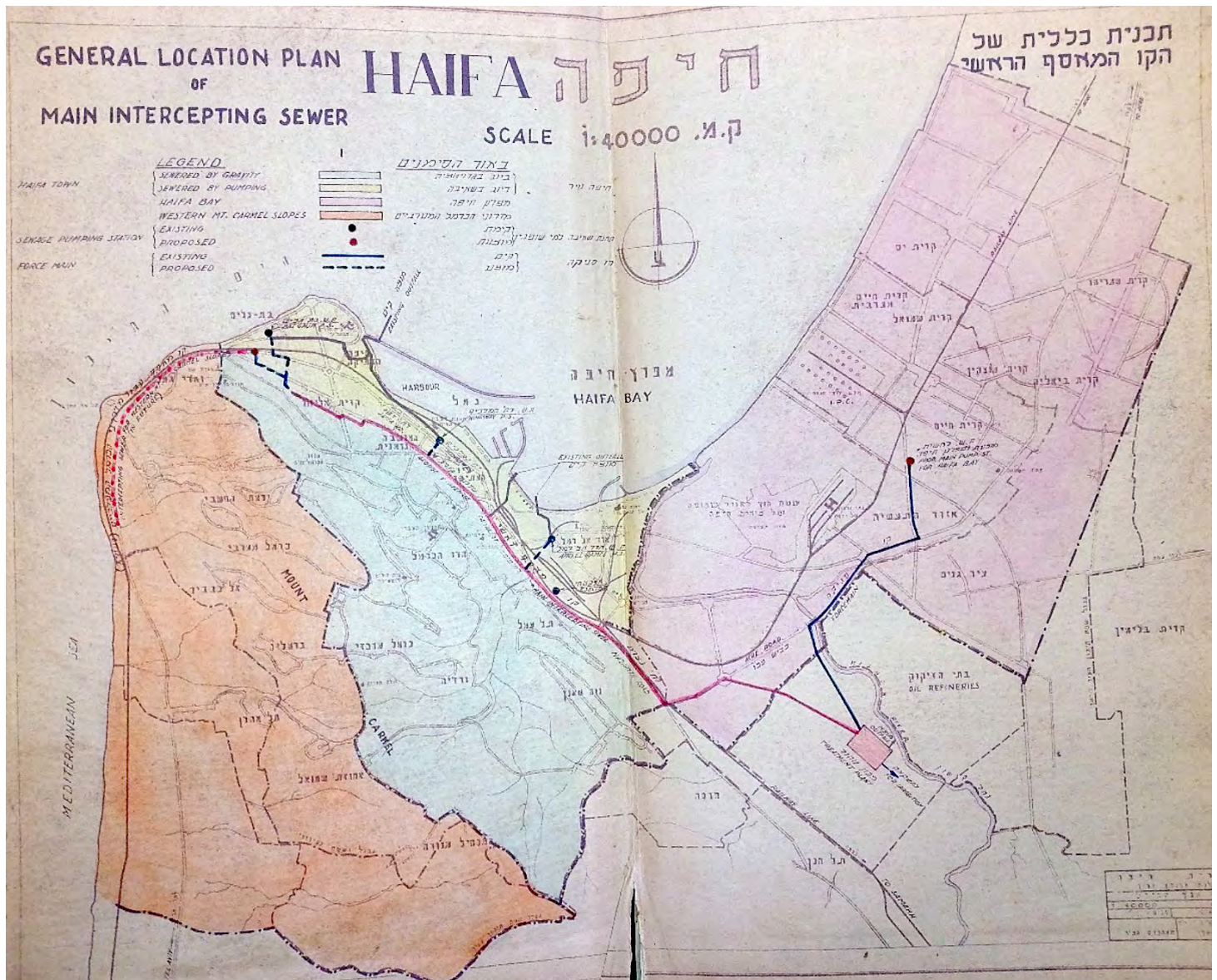
קו המאסף הראשי - תכנון, מ.ה. קלגרמן, דצמבר 1950
